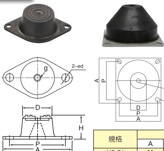
結構圖
