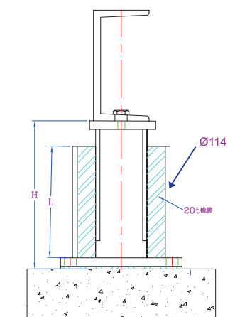
YS-ELS 安裝示意圖
