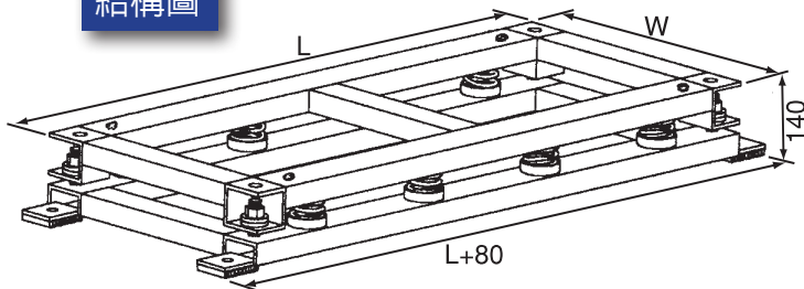
結構圖
